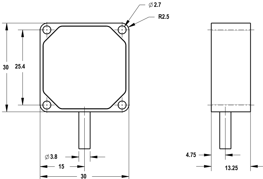
Figura 2. Modello in alluminio
